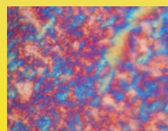
Жидкокристаллические парамагнетики
