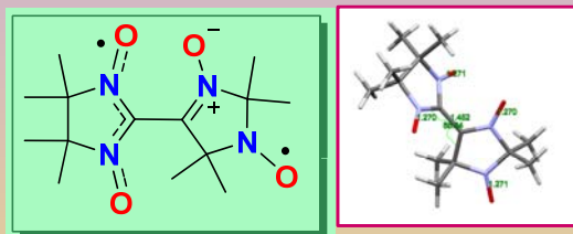
Слабосвязанные гетеродирадикалы
