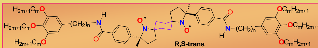
Жидкокристаллические парамагнетики
