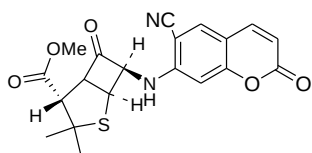
метил (2R,5S,6S)-3,3-диметил-6-[(6-циано-2-оксо-2H-хромен-7-ил)амино]-7-оксо-4-гиа-1-азабицикло[3.2.0]гептан-2-карбоксилат 118f. Получен по методу b) с выходом 65% (0.08 г),
