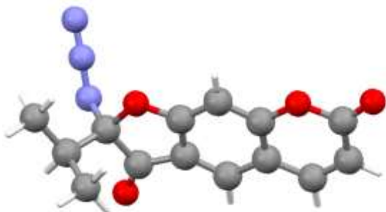
Рис.2. Пространственное строение 2-азидореозелона 20 .
