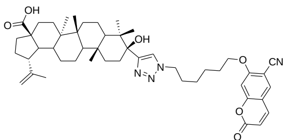
(1 R ,3 a S ,5 a R ,5 b R ,9 S ,11 a R )-9-(1-(6-(6-циано-2-оксо-2 H -хромен-7-илокси)гексил)-1 H -1,2,3-триазол-4-ил)-9-гидрокси-5 a ,5 b ,8,8,11 a -пентаметил-1-(проп-1-ен-2-ил)-изоксагидро-1 H -циклопента[ a ]хризен-3 a -карбоновая кислота 183f. Выход 72% (0.22
