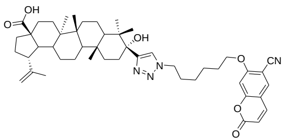
(1 R ,3 a S ,5 a R ,5 b R ,9 R ,11 a R )-9-(1-(6-(6-циано-2-оксо-2 H -хромен-7-илокси)гексил)-1 H -1,2,3-триазол-4-ил)-9-гидрокси-5 a ,5 b ,8,8,11 a -пентаметил-1-(проп-1-ен-2-ил)-изоксагидро-1 H -циклопента[ a ]хризен-3 a -карбоновая
