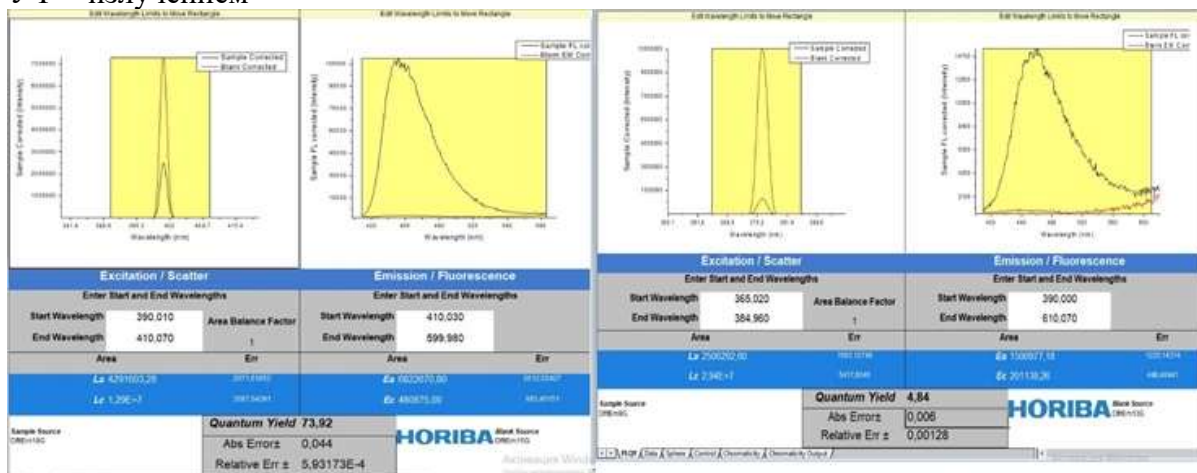
Рис. 3. Сравнение КВ соединений 7 (слева) и 160с (справа) в ДМСО
