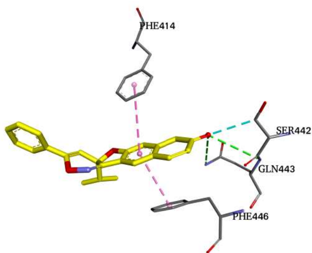
Рисунок 1. 3D взаимодействие лиганда 164a в сайт связывания PDE4B.
