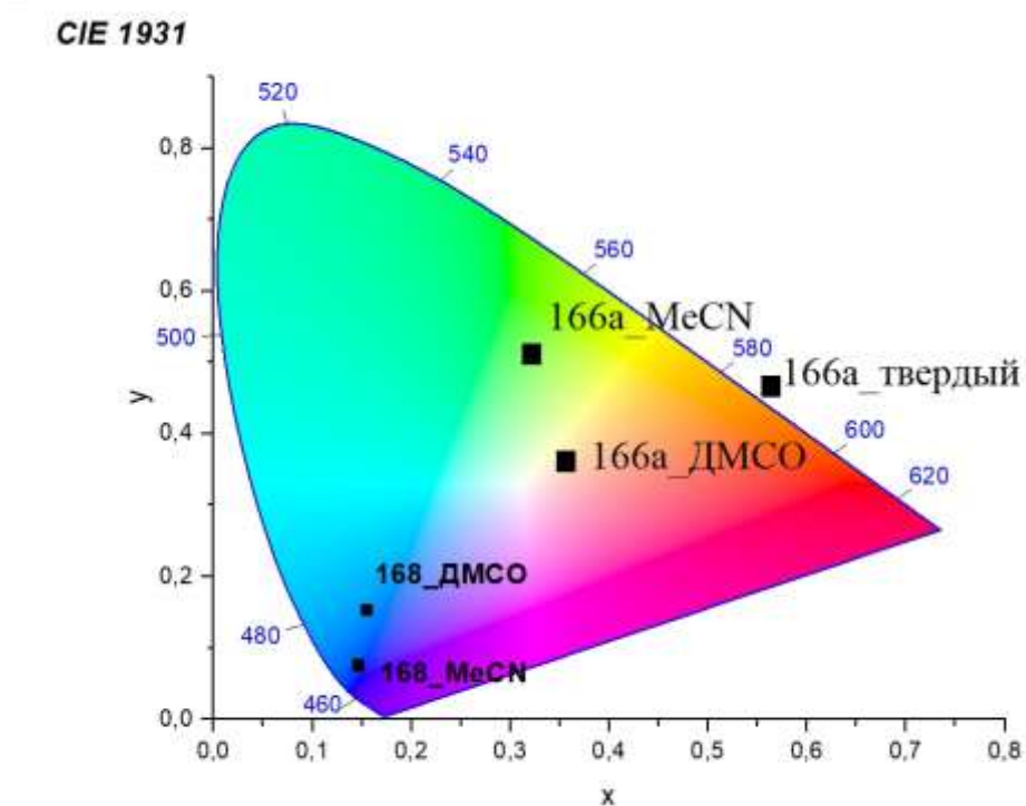
Рис. 8. Диаграмма цветности для соединений 166a и 168
