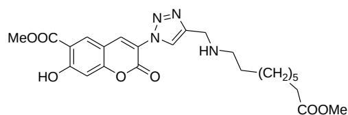
метил 7-гидрокси-3-(4-((9-метокси-9-оксонониламино)метил)-1Н-1,2,3-триазол-1-ил)-2-оксо-2Н-хромен-6-карбоксилат 156а. Раствор 0.05 г (0.19 ммоль) 3-азидопеуртеницина 155 в 10
