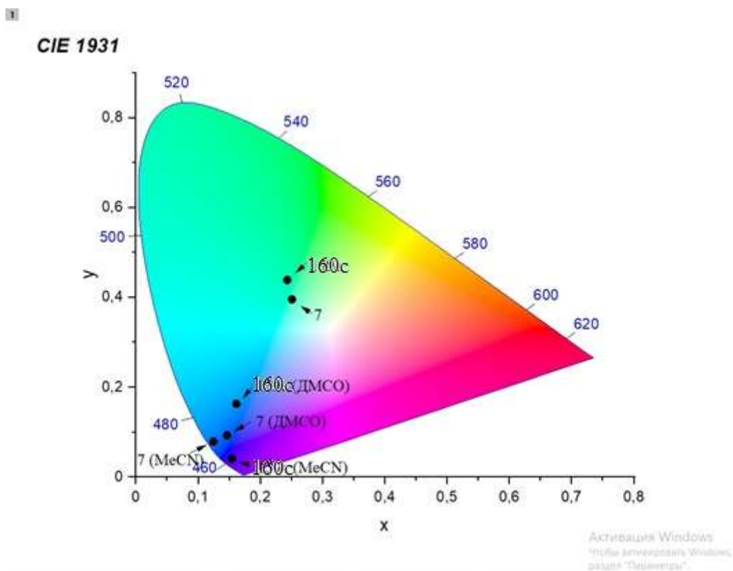
Рис. 7. Диаграмма цветности для соединений 7 и 160c
