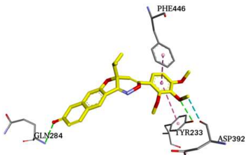
Рисунок 3. 3D взаимодействие лиганда 164c в сайт связывания PDE4B.
