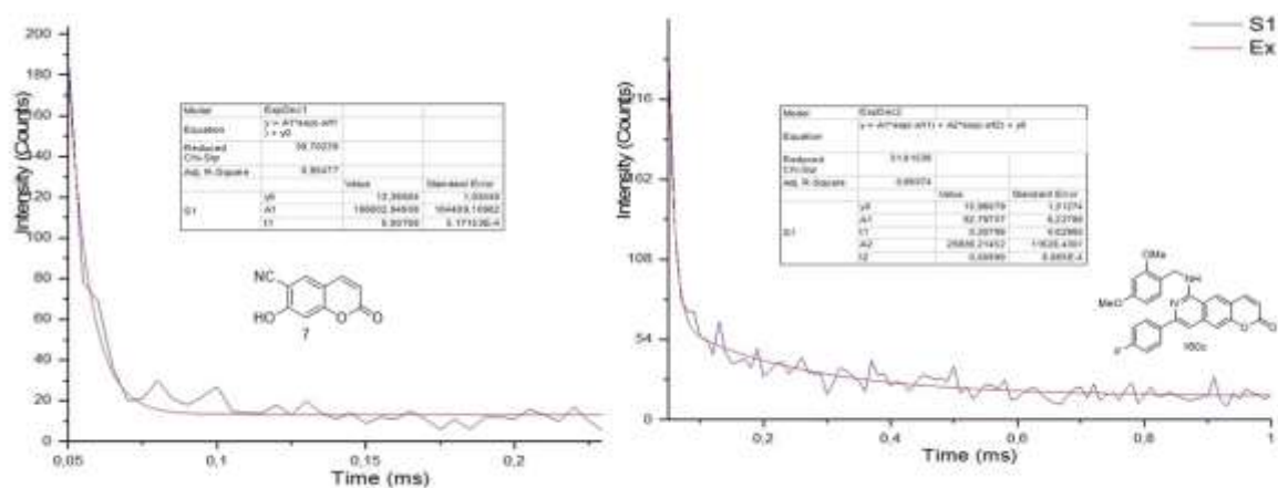
Рис.9. Время жизни соединения 7 и 160с
