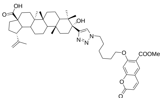
(1R,3 a S,5 a R,5 b R,11 a R)-9-гидрокси-9-(1-(6-(6-метоксикарбонил)-2-оксо-2H-хромен-7-илокси)гексил)-1H-1,2,3-триазол-4-ил)-5 a ,5 b ,8,8,11 a -пентаметил-1-(проп-1-ен-2-ил)-изоксагидро-1H-циклопента[а]хризен-3 a -карбоновая кислота 183d. Выход 60% (0.198 г),
