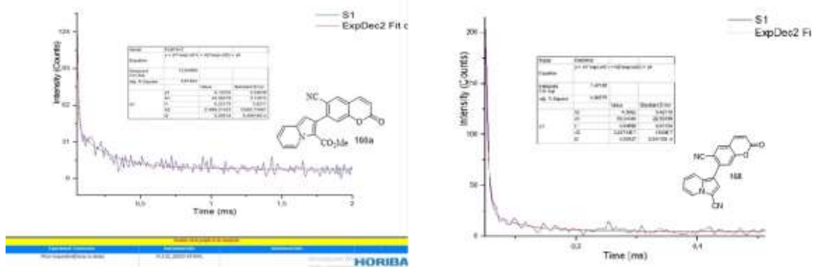
Рис.10. Время жизни соединений 166a и 168
