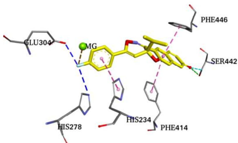
Рисунок 3. 3D взаимодействие лиганда 164c в сайт связывания PDE4B.
