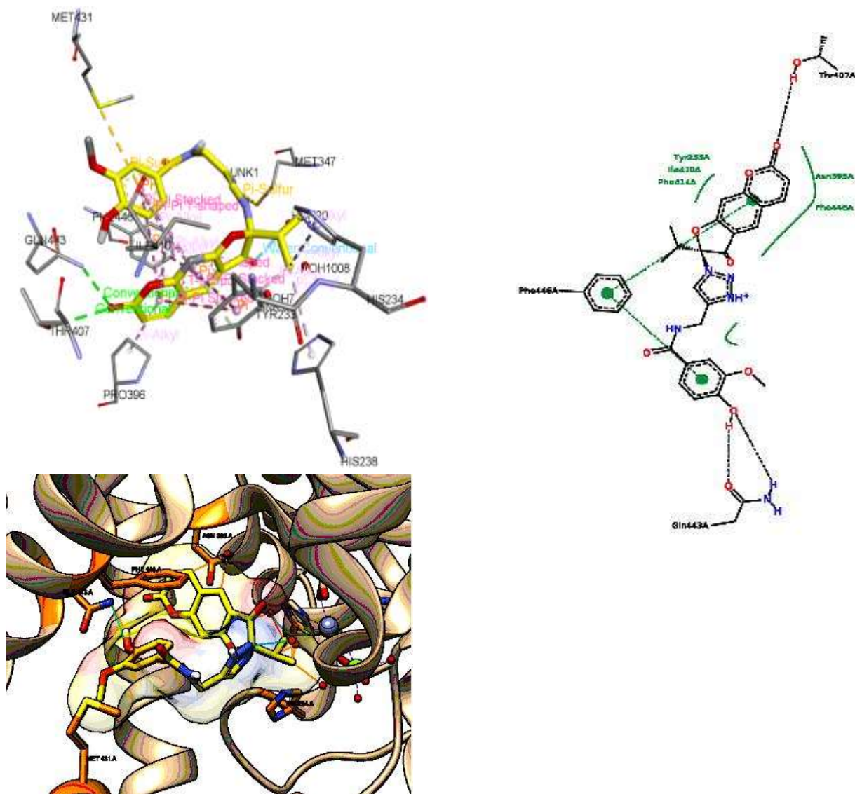
Рисунок 1. 3D взаимодействие лиганда 74 в сайт связывания PDE4B.
